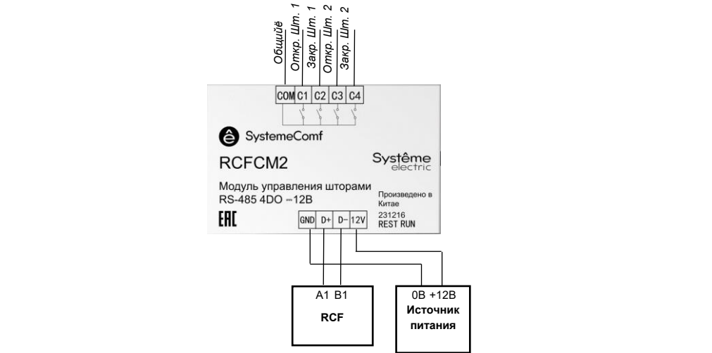
Схема подключения
